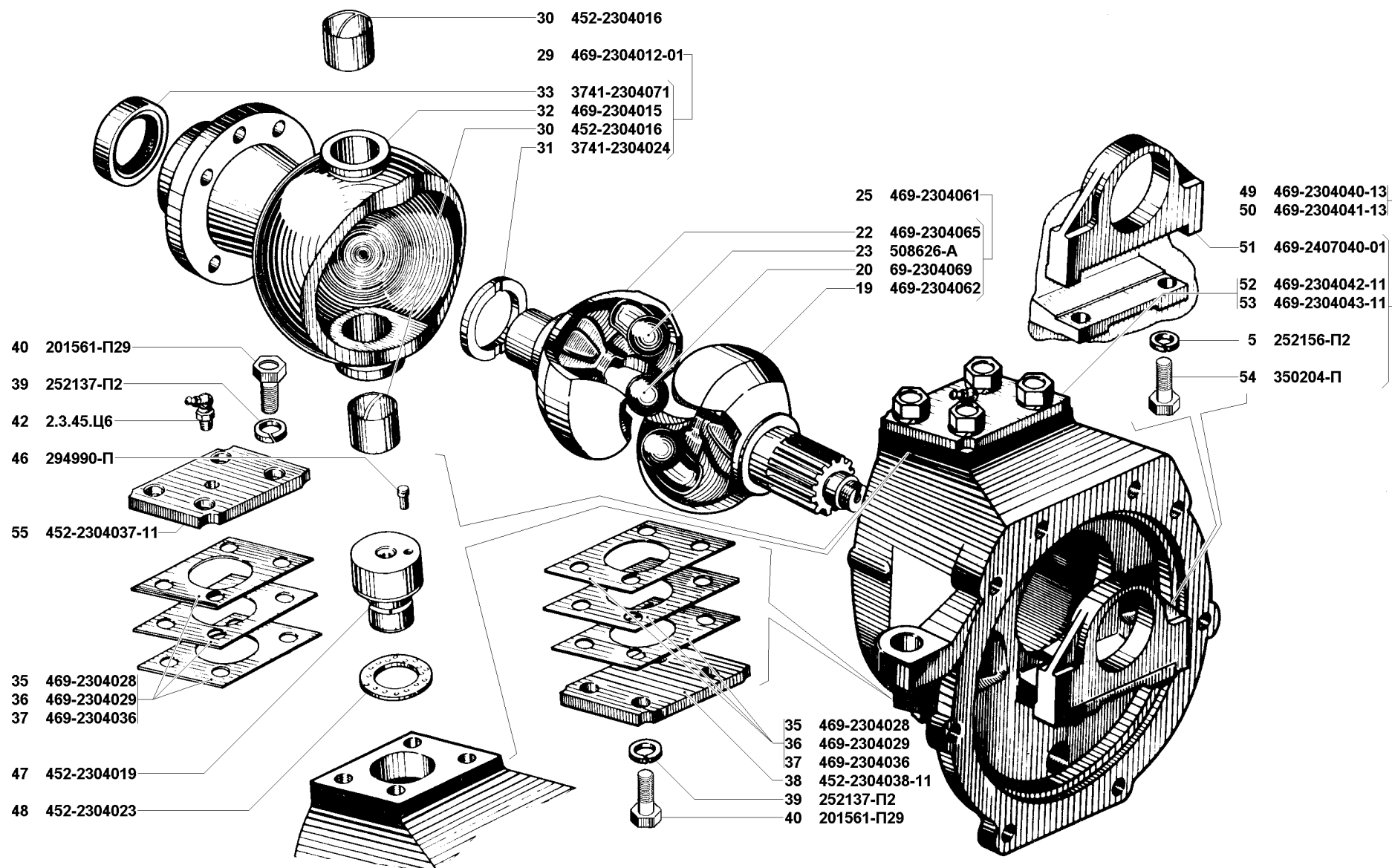
Рис. 70. Кулаки поворотные (2304)/3
